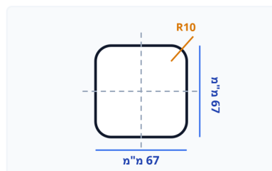
שקע יחיד (67×67)
